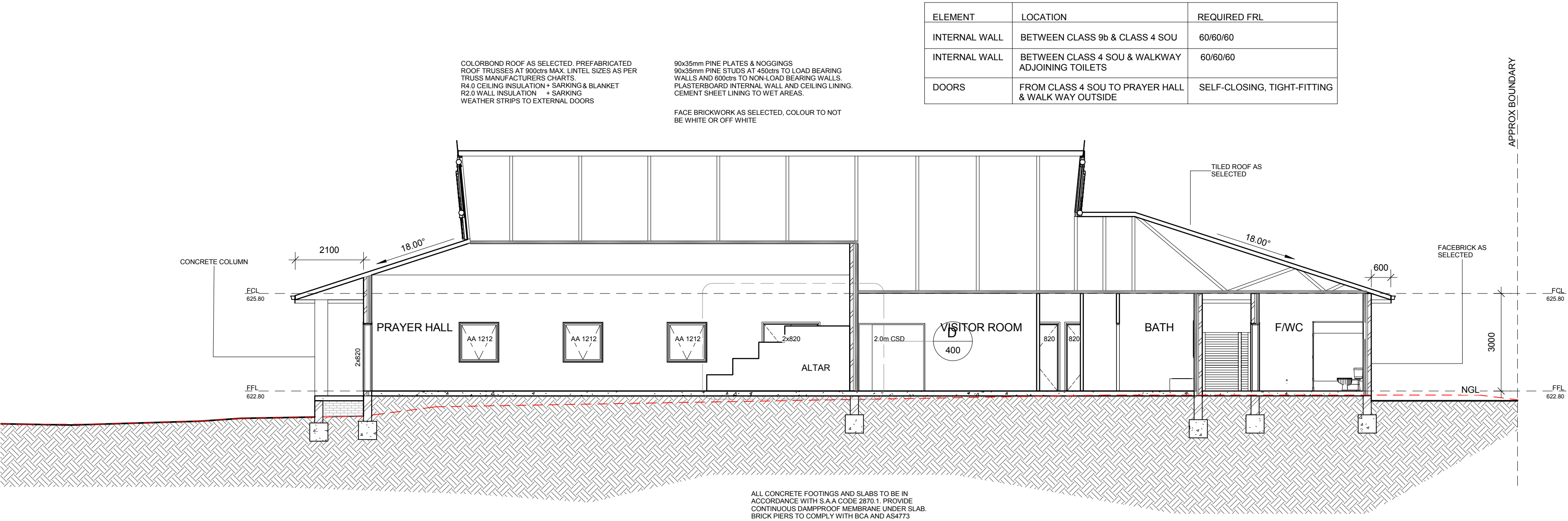
Section C-C 1 : 100
