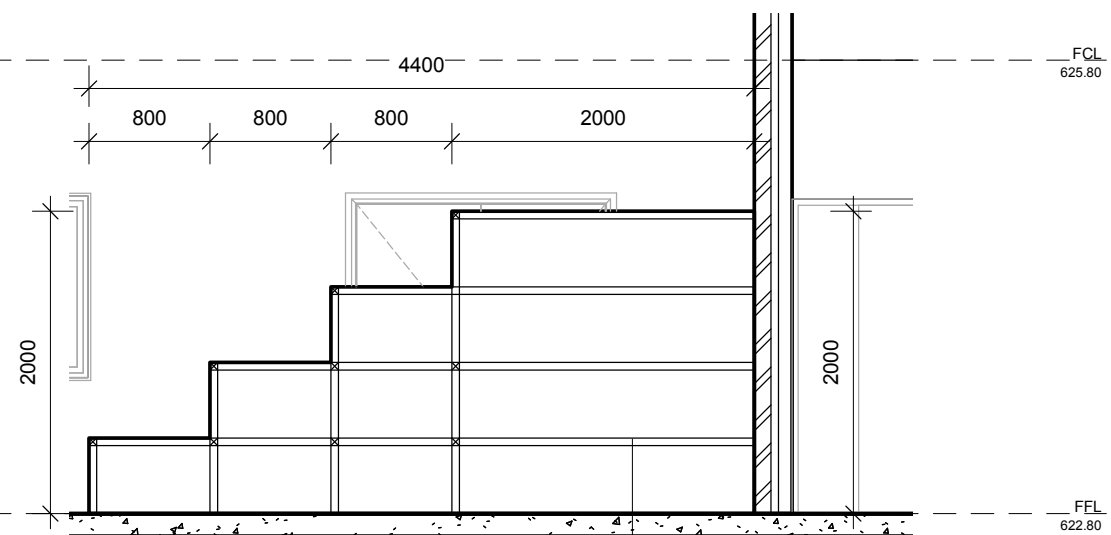
Section D-D 1 : 50
